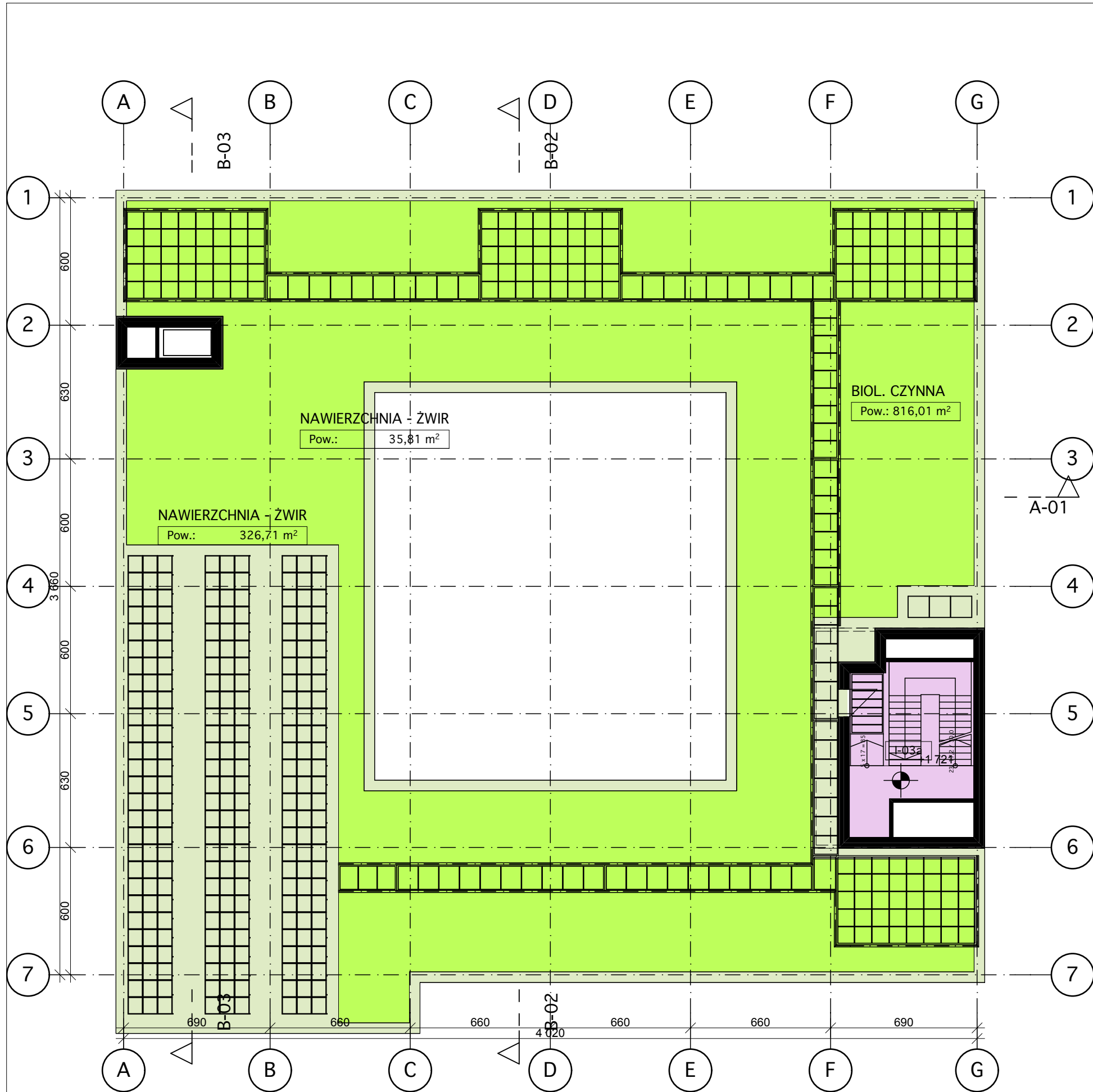
Rzut poziomu kondygnacji technicznej
