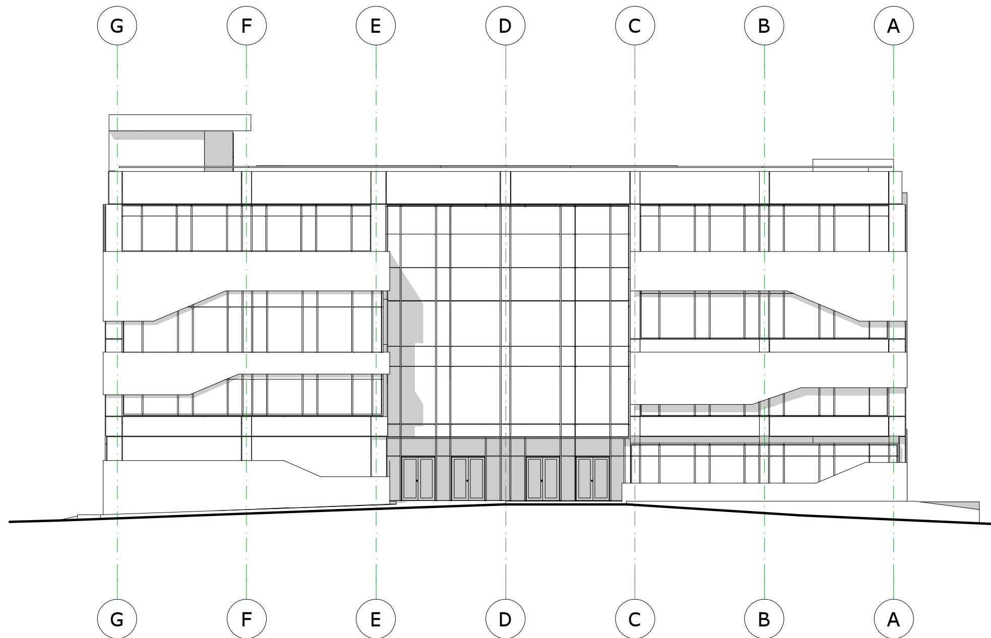
Elewacja Płn.-Wsch.
