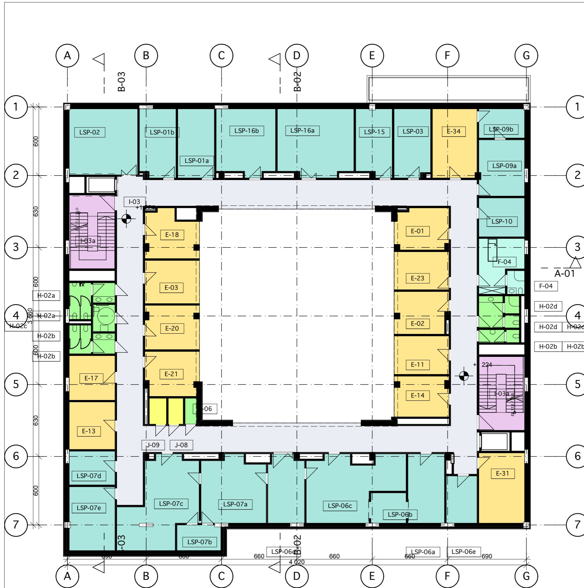
Rzut poziomu +3
